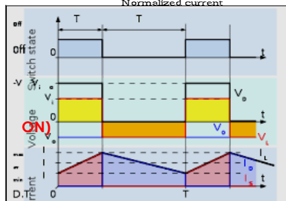
CCM mode
