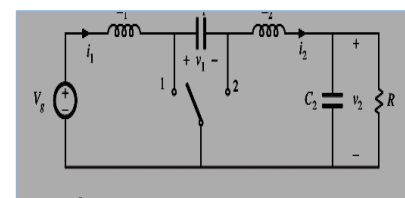
CUK Converter
