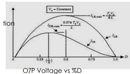
O/P Voltage vs %D
