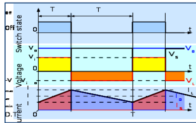
CCM mode
